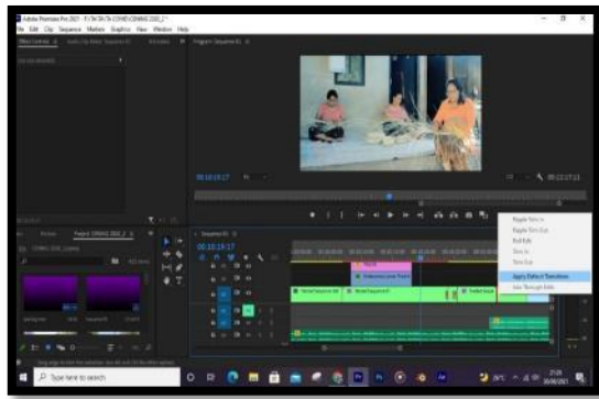
Gambar 4.4 Efek Transisi
