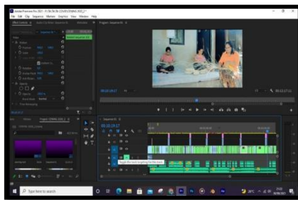
Gambar 4.3 Pemotongan Video
