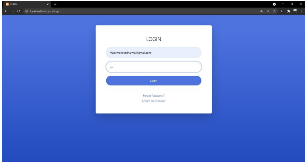
Gambar 1. Halaman Login
