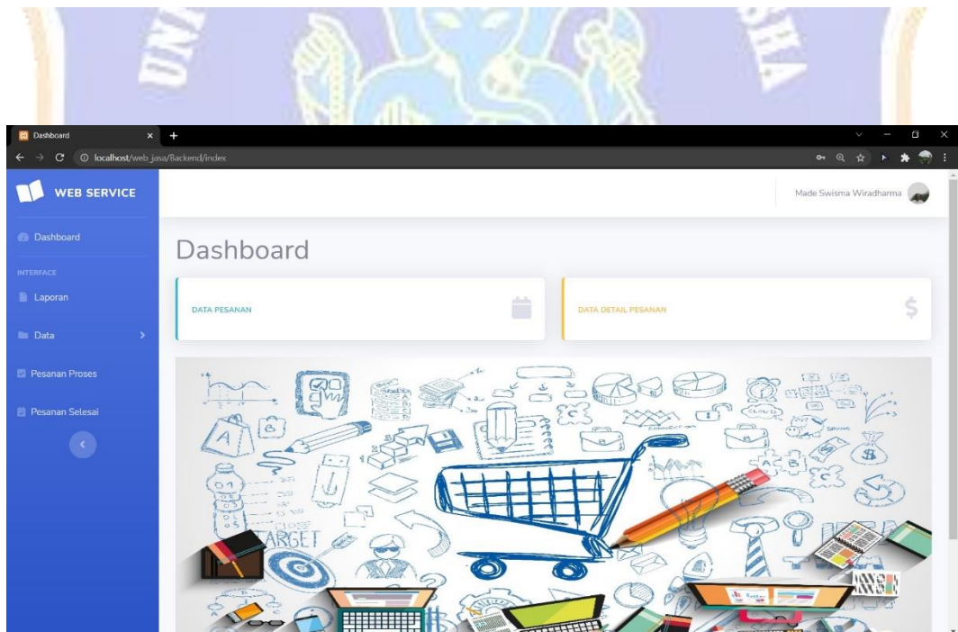
Gambar 2. Login Sukses
