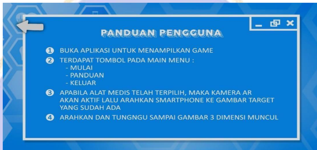
Gambar 7. Tampilan Panduan.
