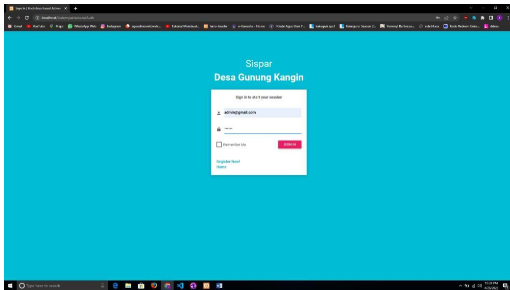
Gambar 1 Halaman Login
