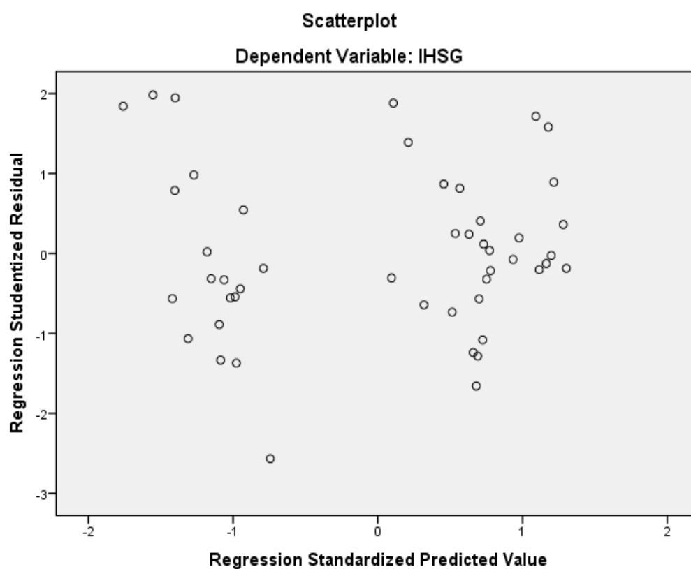
Gambar 4.2 Hasil Uji Heteroskedastisitas
