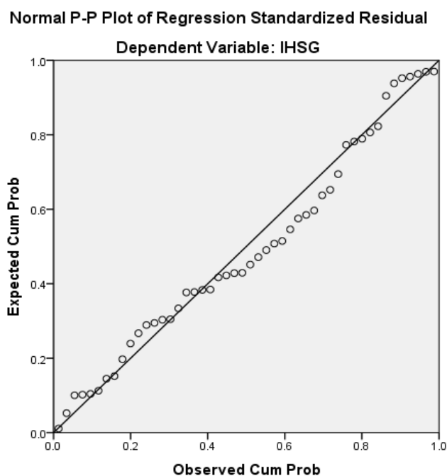
Gambar 4.1 Hasil Uji Normalitas (Sumber: Data Diolah, 2019)
