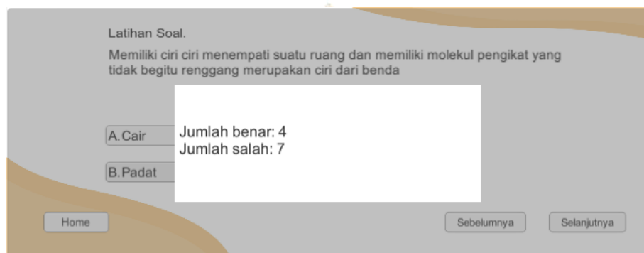
Gambar 17 Hasil Akhir
