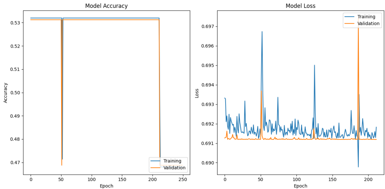
Grafik Epoch 250 Neuron 128
