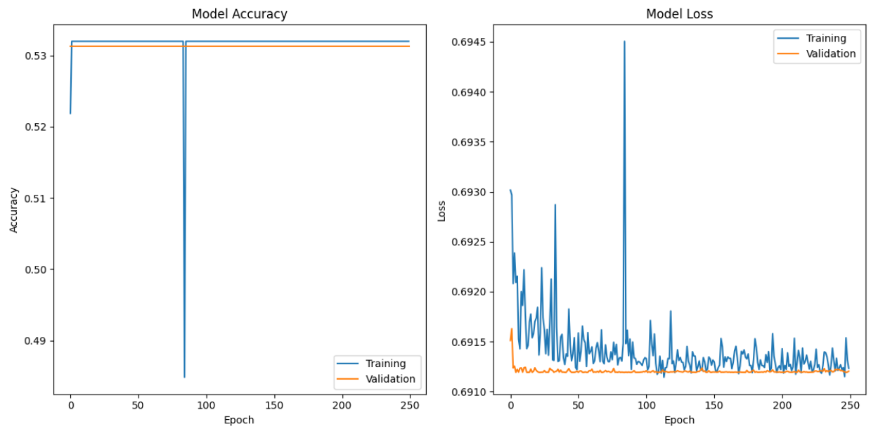
Grafik Epoch 250 Neuron 256
