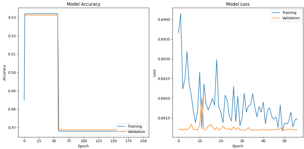
Grafik Epoch 200 Neuron 128
