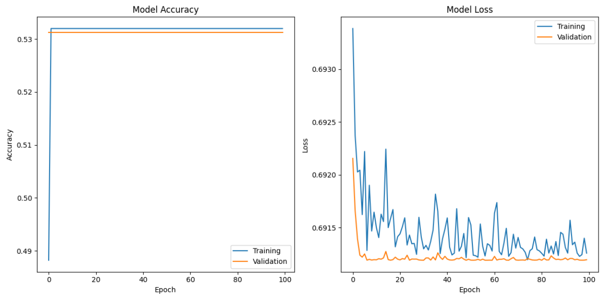
Grafik Epoch 100 Neuron 64
