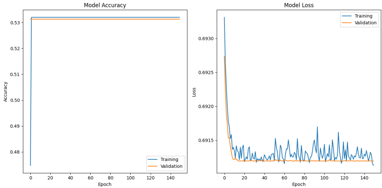
Grafik Epoch 150 Neuron 128
