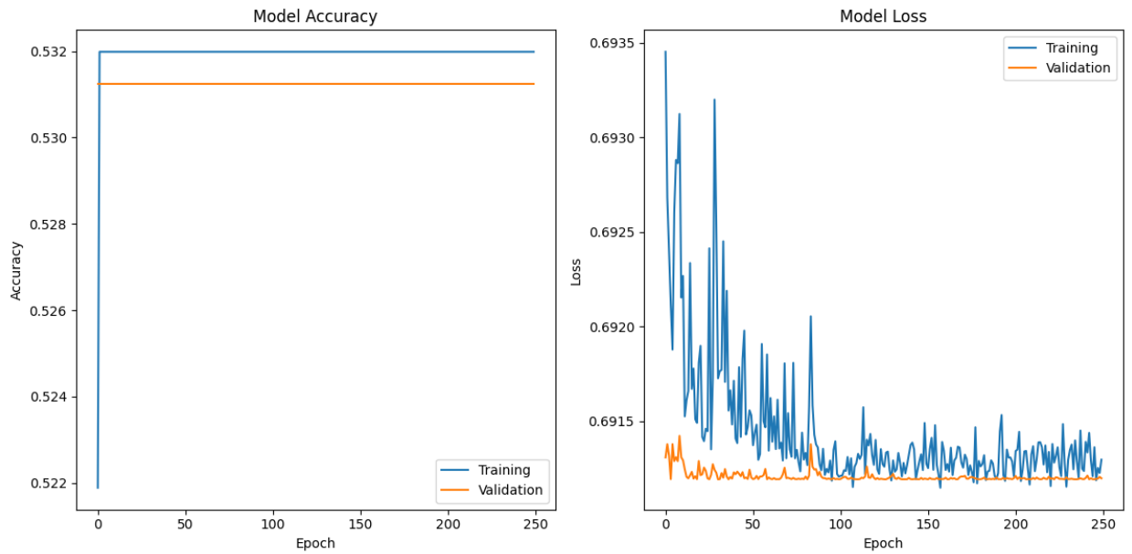
Grafik Epoch 250 Neuron 64
