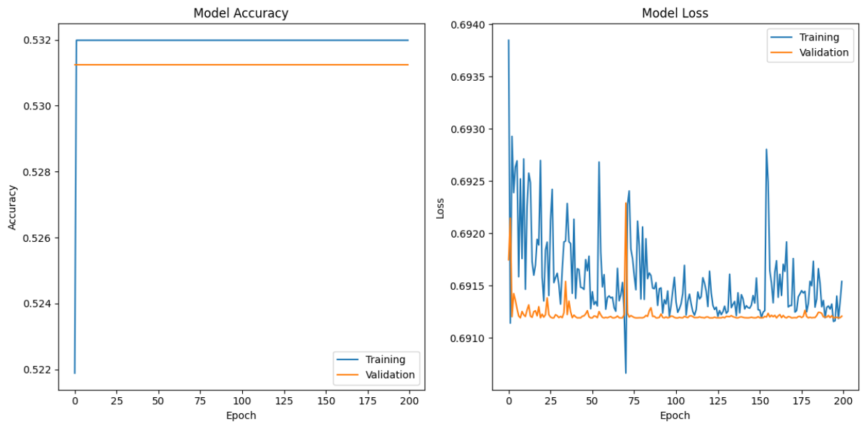
Grafik Epoch 200 Neuron 256
