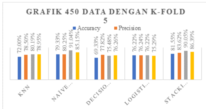
Lampiran 1 Grafik Pengujian Fold 5
