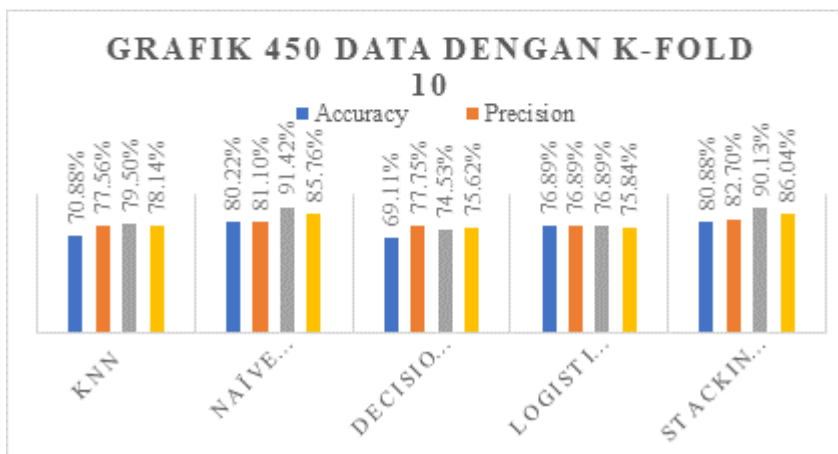
Lampiran 2 Grafik Pengujian Fold 10
