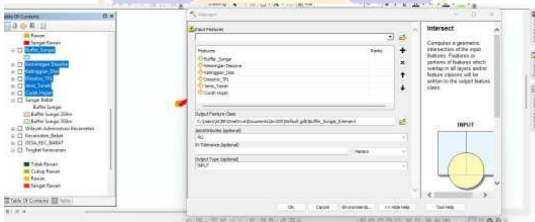
Gambar Proses Overlay 6 Parameter Kerawanan Banjir
