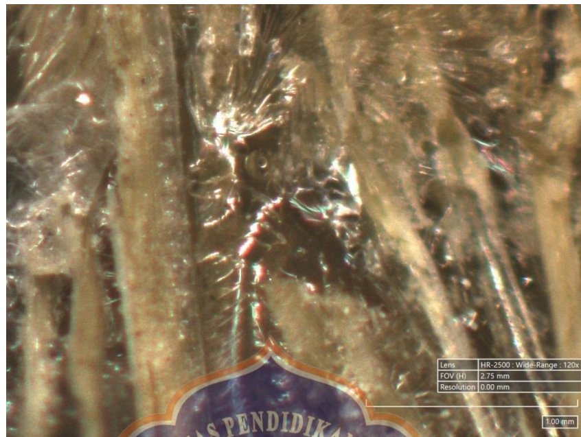
Pola patahan Fraksi Volume 5% Perbesaran 100x
