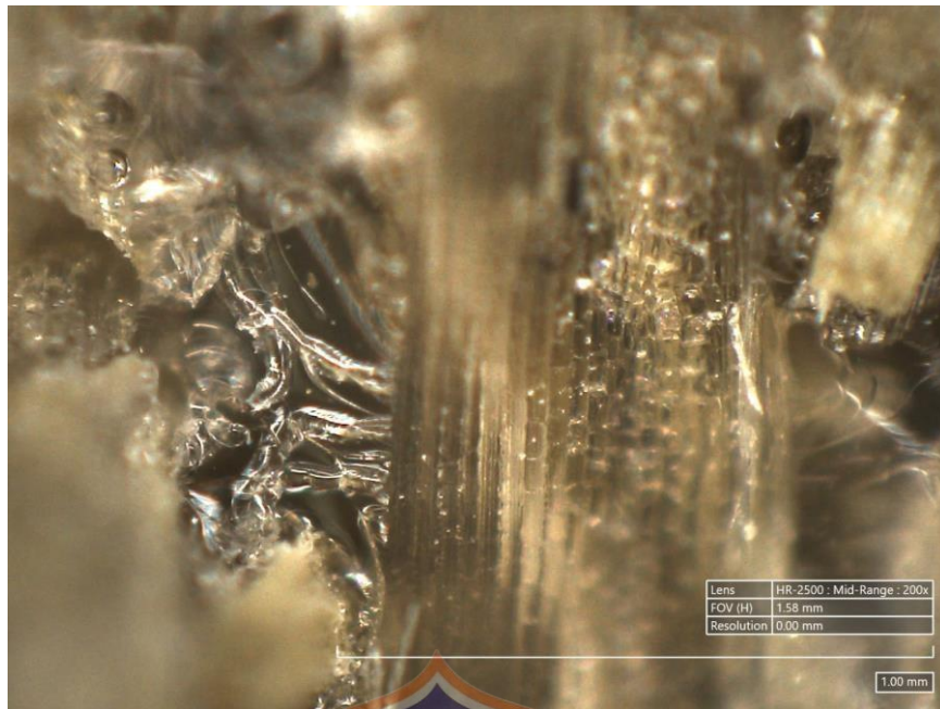
Pola patahan Fraksi Volume 5% Perbesaran 200x
