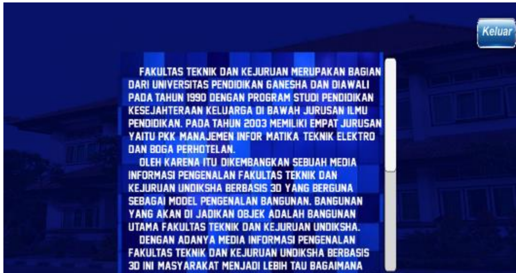
Gambar 5. Menu Tentang.
