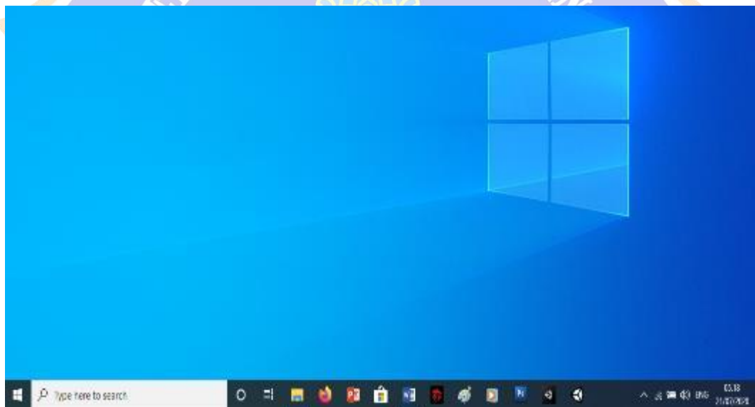
Gambar 6. Menu Keluar
