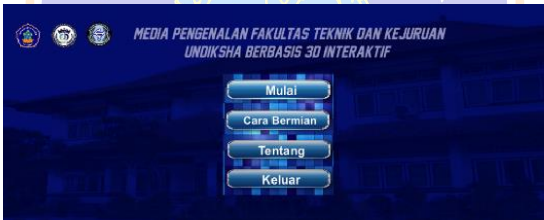
Gambar 2. Menu Utama.
