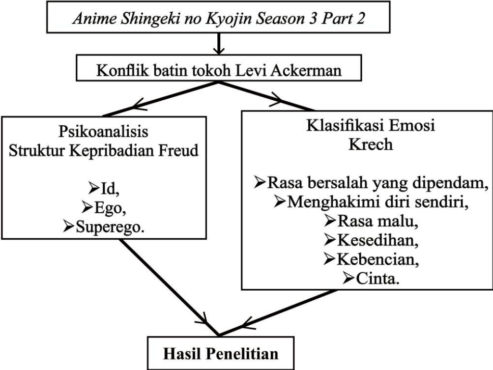
Gambar 01. Kerangka Berpikir
