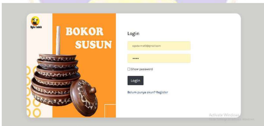
Gambar 3 Login Pelanggan
