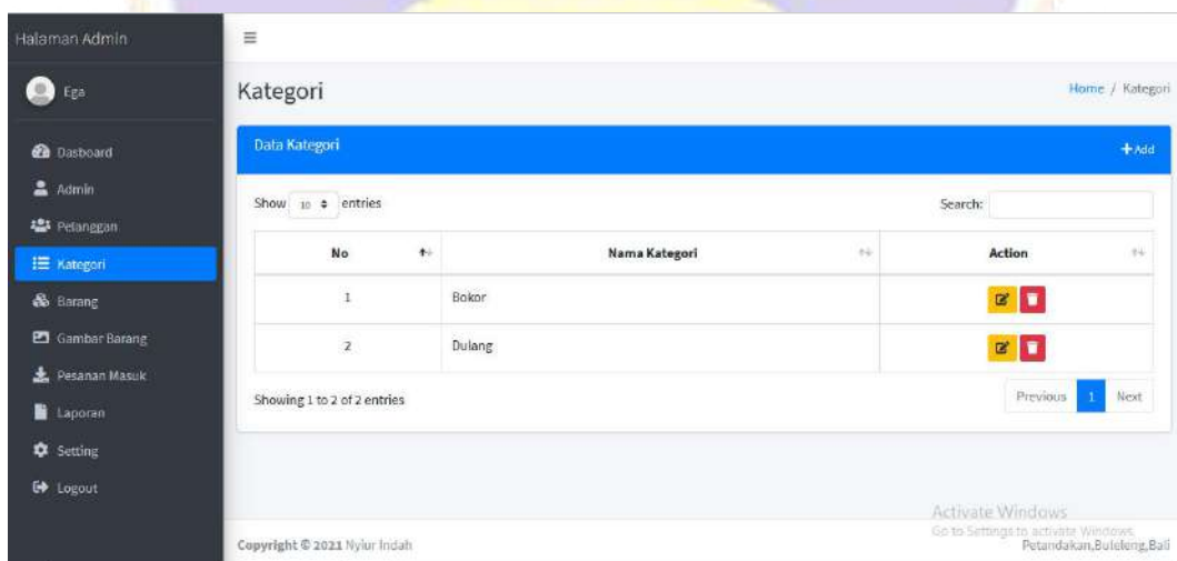
Gambar 12 Halaman Kategori
