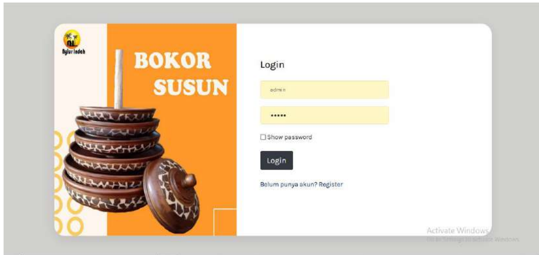
Gambar 1 Login admin
