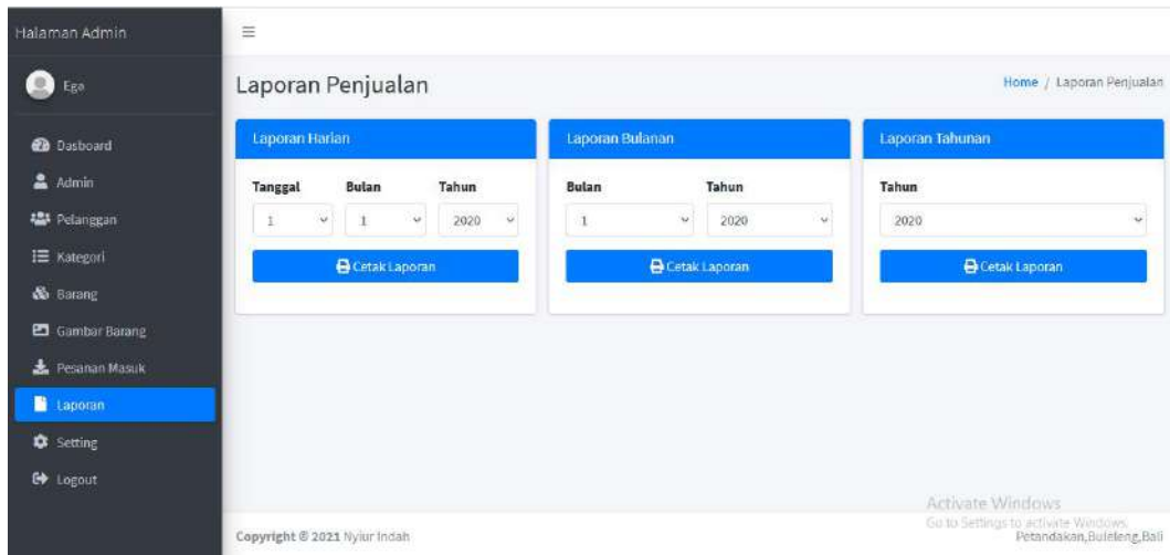
Gambar 31 Cetak Laporan
