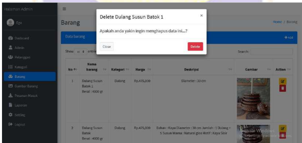
Gambar 24 Hapus Barang
