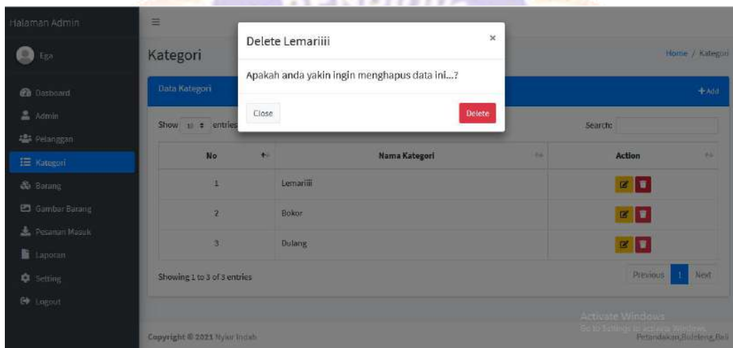
Gambar 17 Hapus Kategori
