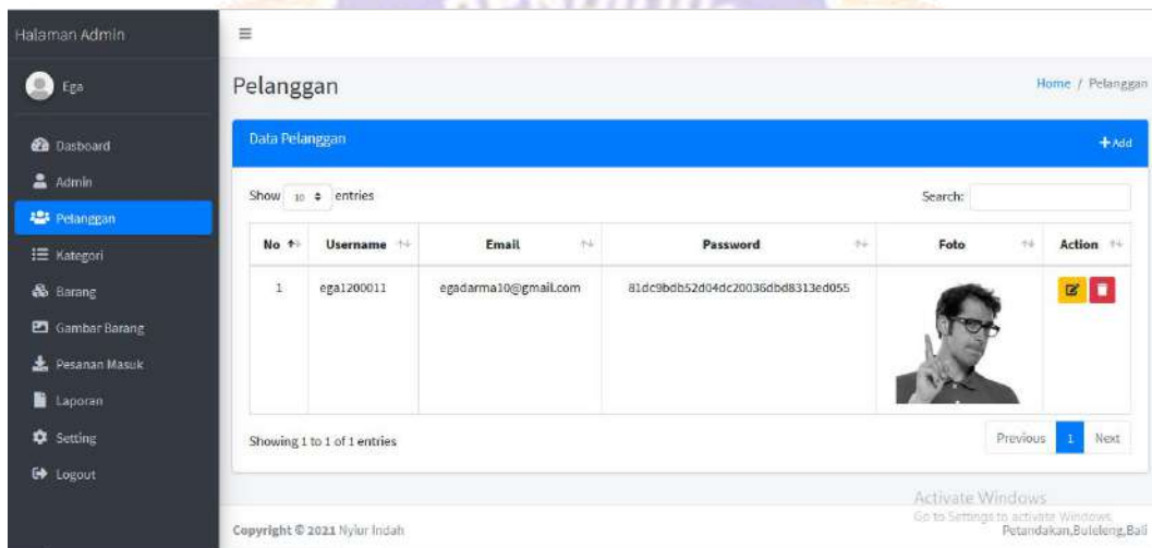
Gambar 5 Pelanggan
