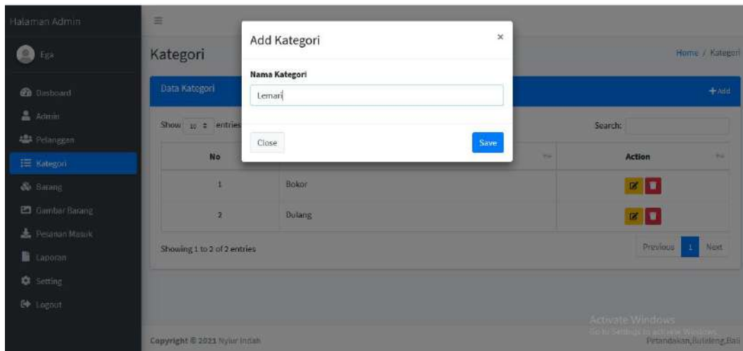
Gambar 13 Tambah Kategori
