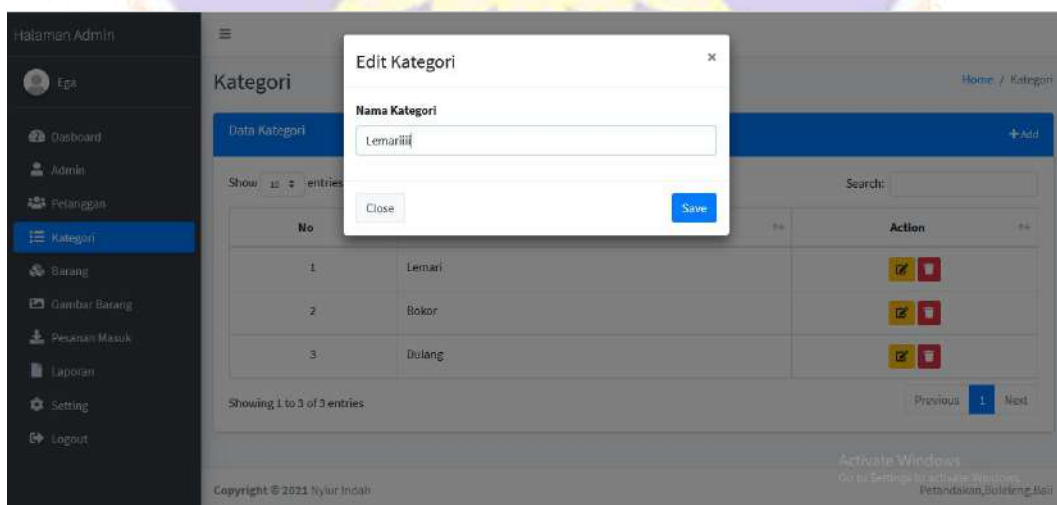
Gambar 15 Edit Kategori
