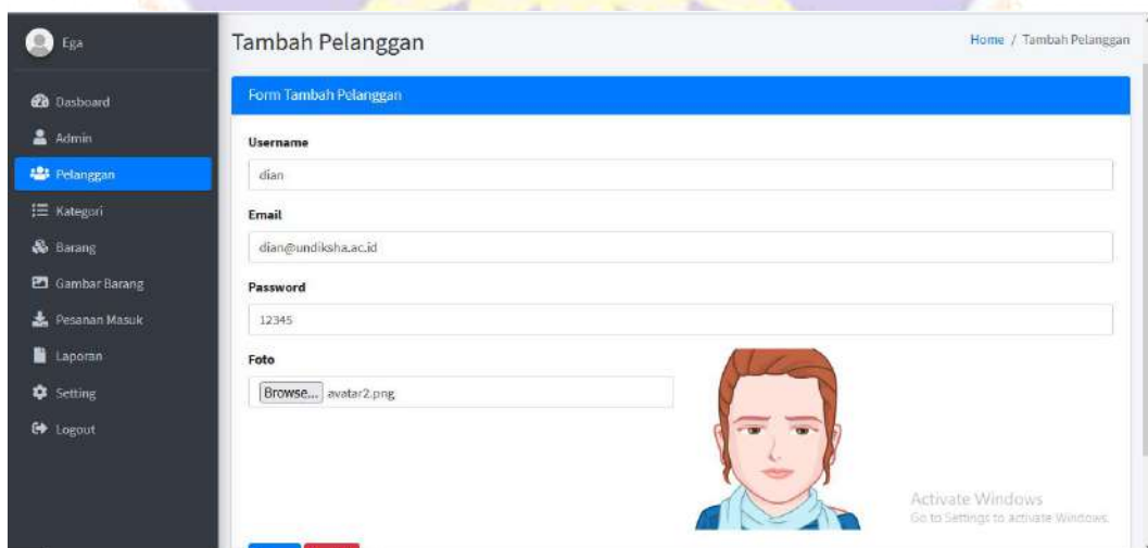
Gambar 6 Tambah Pelanggan
